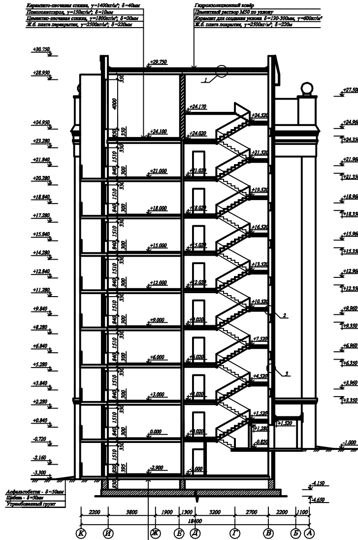
Разрез 1-1
