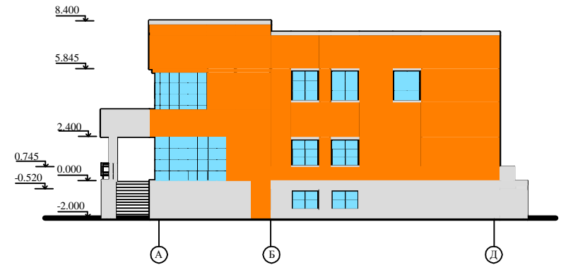
ФАСАД А-Д
