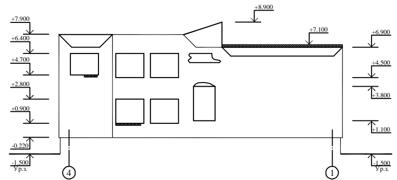
Фасад 1-4 до реконструкции
