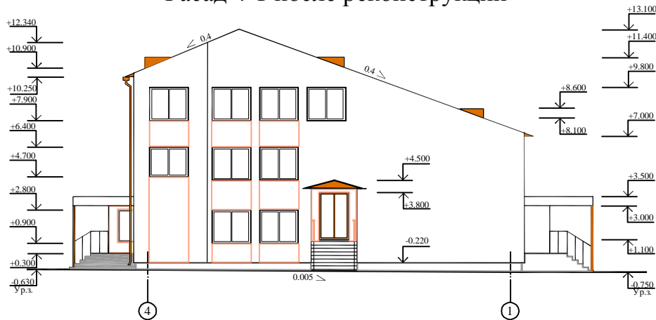
Фасад 1-4 после реконструкции
