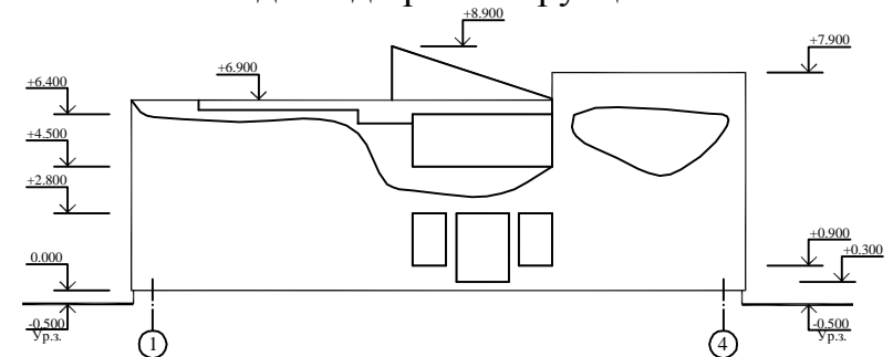
Фасад 1-4 до реконструкции
