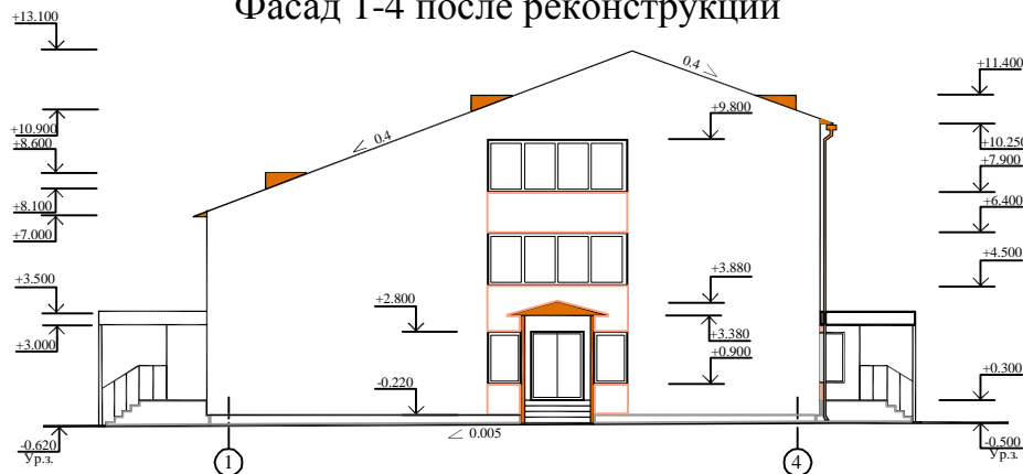
Фасад 1-4 после реконструкции
