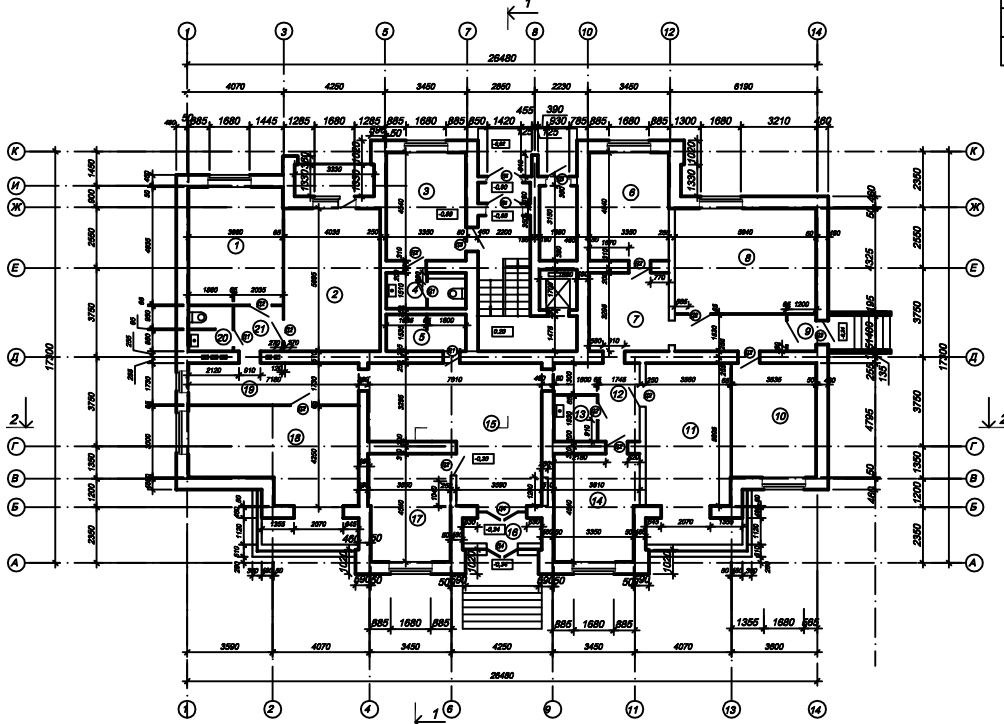
План першого поверху в осях 1-14
